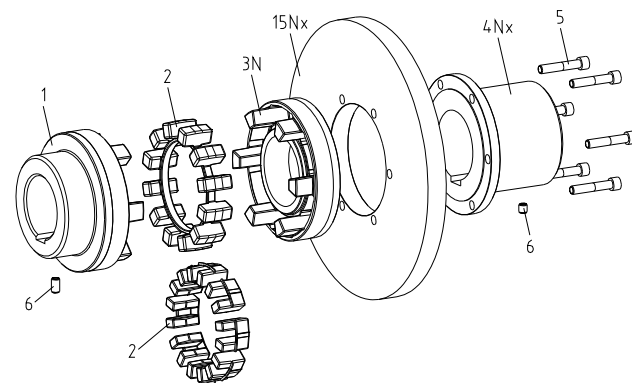
rysunek 16: POLY-NORM® AR-SB
