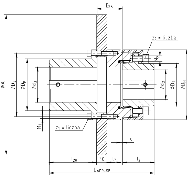
rysunek 6: POLY-NORM® ADR-SB
