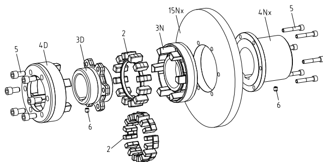
rysunek 14: POLY-NORM® ADR-SB
