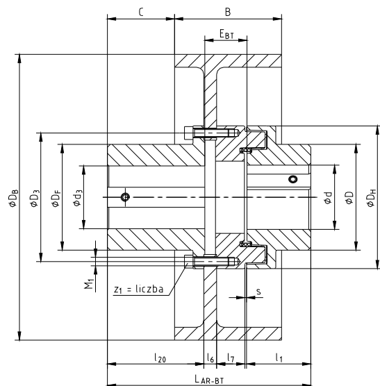
rysunek 7: POLY-NORM® AR-BT
