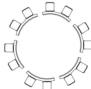
rysunek 23: ułatwienie w montażu łącznika elastycznego (od rozmiaru 75)
