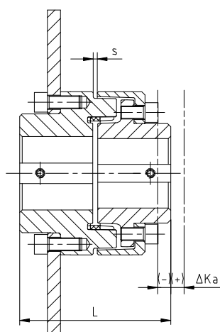
odchyłka osiowa
