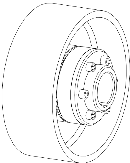
POLY-NORM® ADR-BTA, AR-BTA, ADR-BT oraz AR-BT
