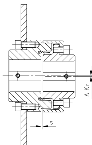
odchyłka promieniowa
