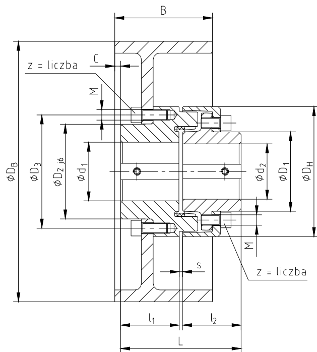
rysunek 1: POLY-NORM® ADR-BTA
