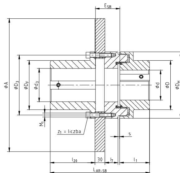
rysunek 8: POLY-NORM® AR-SB
