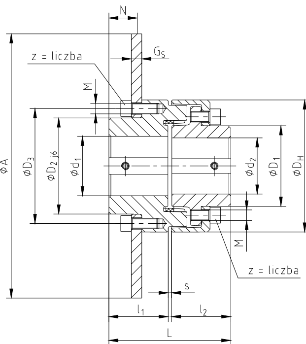
rysunek 2: POLY-NORM® ADR-SBA
