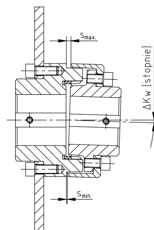
odchyłka kątowa
