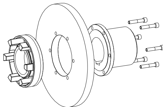
rysunek 19: montaż tarczy hamulcowej (typ SB oraz BT)
