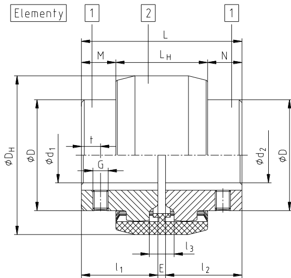
rysunek 3: BoWex® wykonanie M
