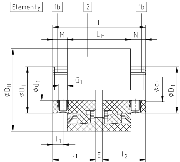
rysunek 2: BoWex® junior M sprzęgło 3-częściowe
