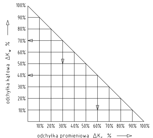
rysunek 11: połączenie odchyłek
