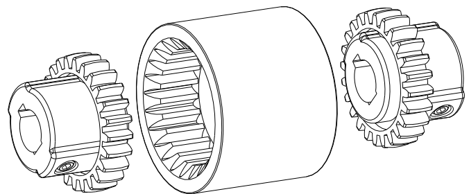
wykonanie sprzęgło junior M (3-częściowe)
