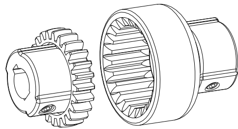
wykonanie sprzęgło junior (2-częściowe)
