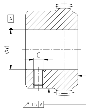
rysunek 9: współśrodkowość i osiowość obróbki
