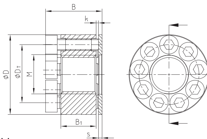
nakrętka zaciskowa
