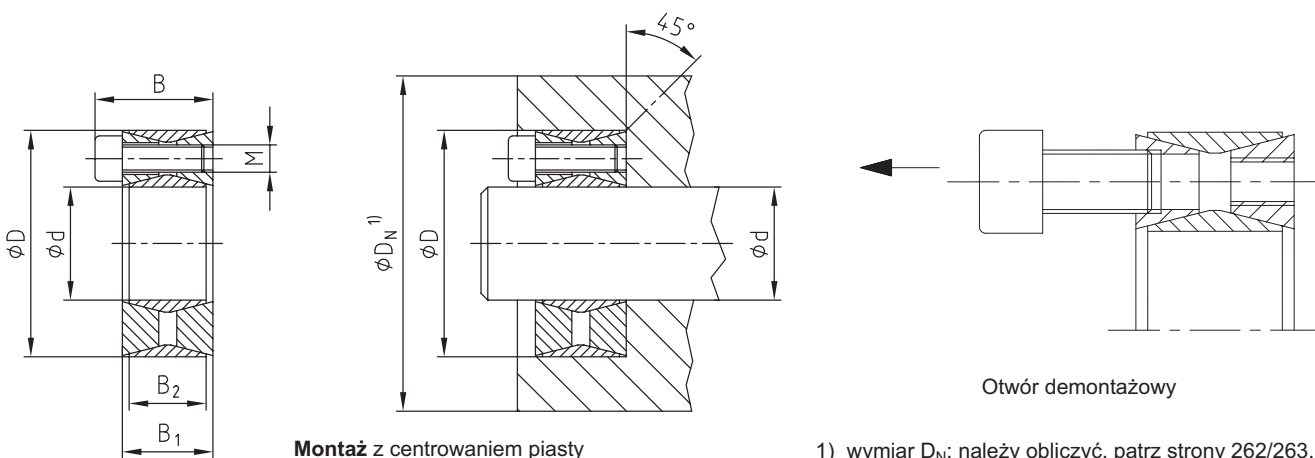
Montaż z centrowaniem piasty
