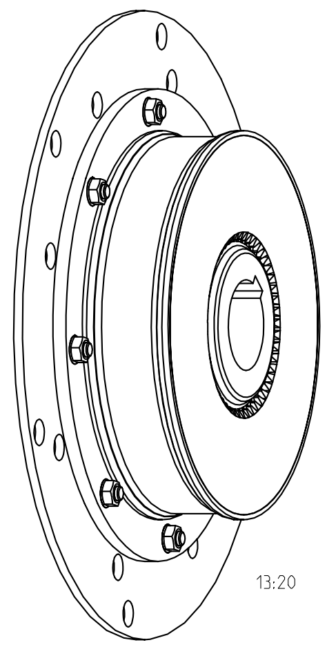
Passfedernut nach DIN 6885
