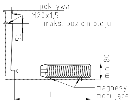
rysunek 6: sposób montażu – TEHM
