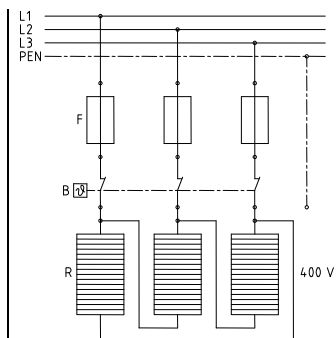
rysunek 12: schemat połączeń z termostatem – 400 V \star
