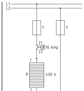
rysunek 8: schemat połączeń z termostatem – 400 V
