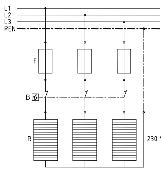
rysunek 11: schemat połączeń z termostatem – 230 V \star
