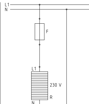
rysunek 9: schemat połączeń bez termostatu – 230 V
