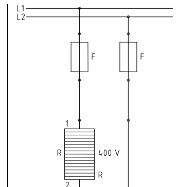
rysunek 10: schemat połączeń bez termostatu – 400 V
