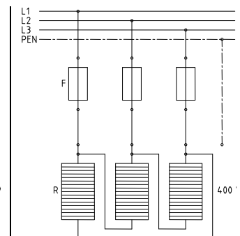
rysunek 14: schemat połączeń bez termostatu – 400 V \triangle
