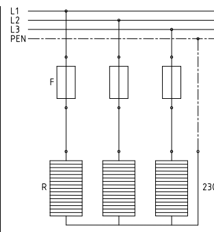
rysunek 13: schemat połączeń bez termostatu – 230 V \star
